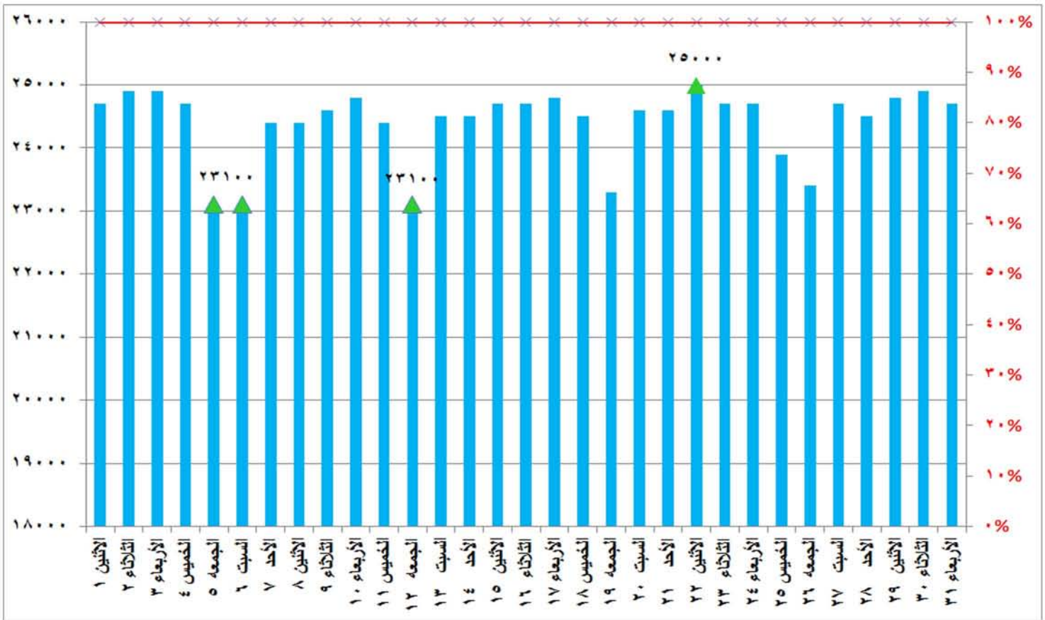
شكل (٥) قدرات الانتاج المتاحة ونسبتها للحمل الأقصى خلال شهر يناير ٢٠١٨
