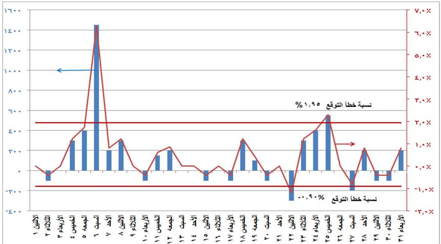
شكل (١٠) الفرق بين الحمل الأقصى المتوقع والمسجل فعلياً ونسبة الفرق إلى الحمل المسجل فعلياً خلال شهر يناير ٢٠١٨
