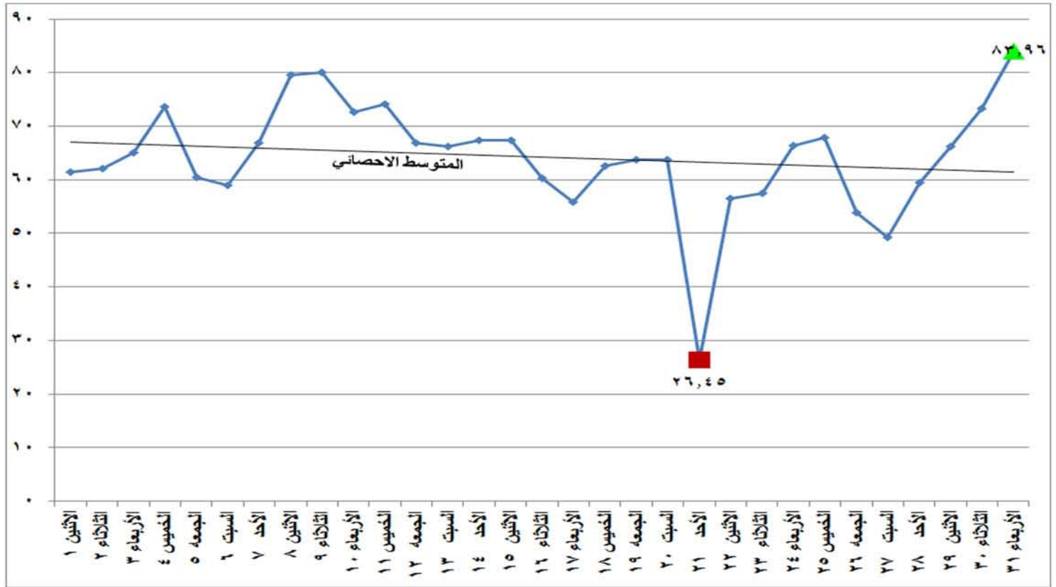
شكل (١٩) الطاقة الكهربائية المنتجة من المازوت خلال شهر يناير ٢٠١٨
