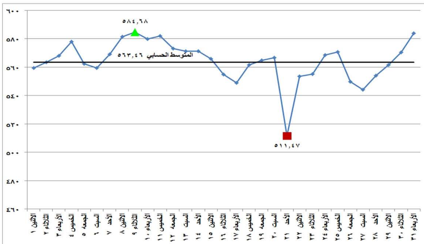
شكل (١٤) معامل انبعاثات غاز ثاني اكسيد الكربون المكافئ على مدى شهر يناير ٢٠١٨
