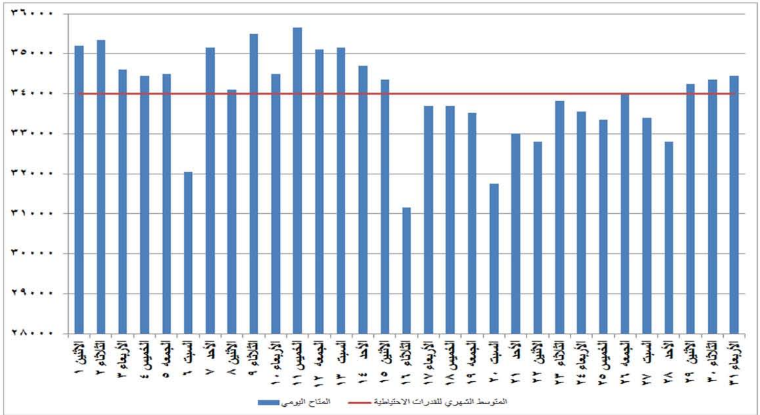
شكل (٢٧) القدرات المتاحة يوميا والمتوسط الشهري للقدرة الاحتياطية خلال شهر يناير ٢٠١٨
