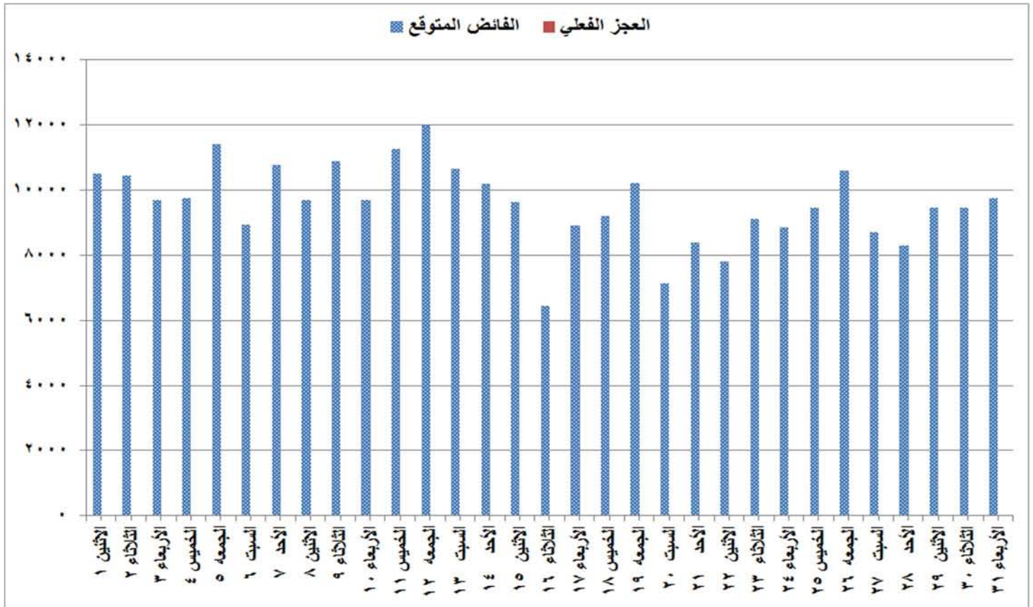
شكل (٧) الفائض والعجز المتوقع للقدرات خلال شهر يناير ٢٠١٨
