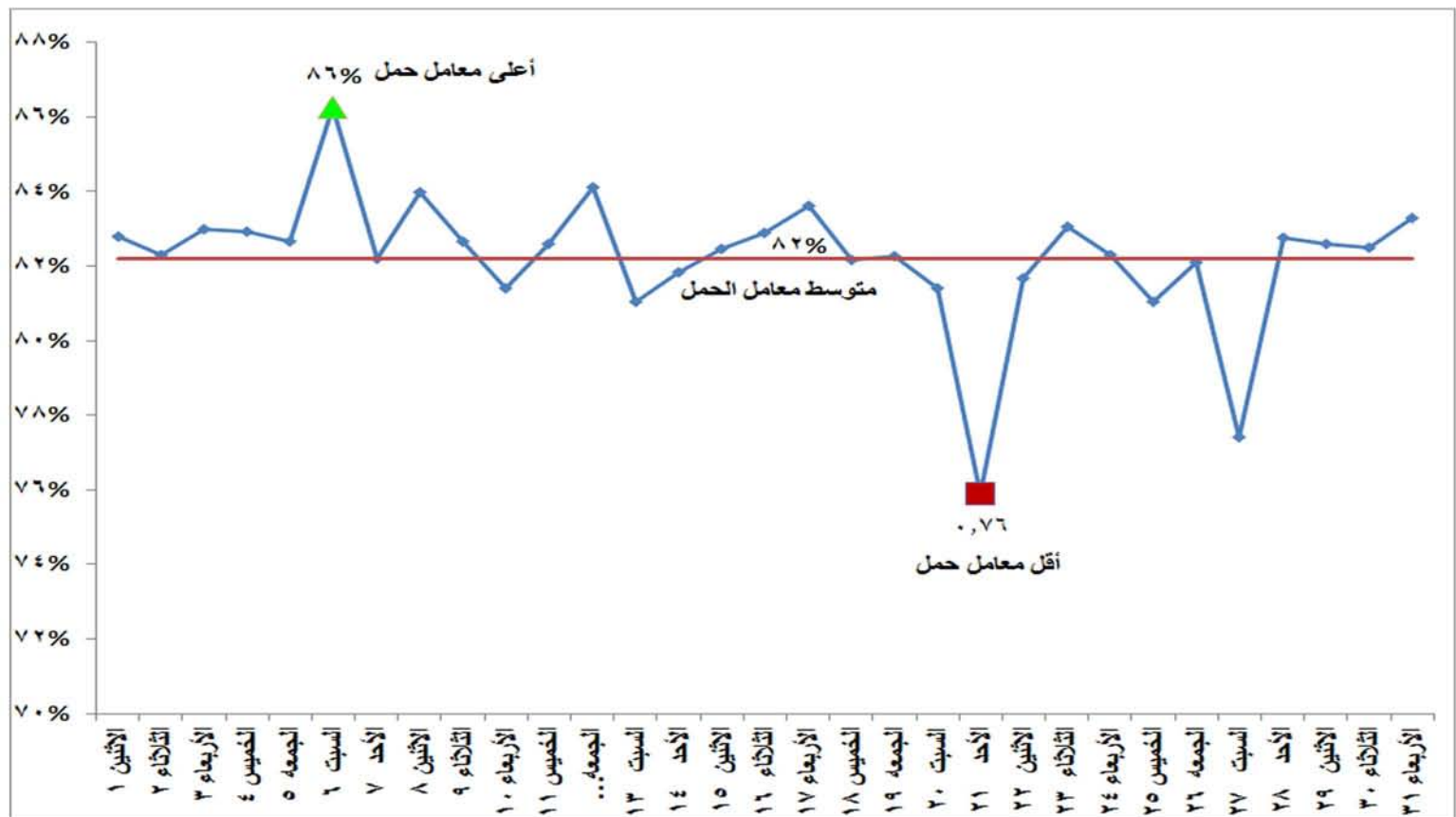
شكل (١٢) إجمالي معامل الحمل لوحدات الانتاج خلال شهر يناير ٢٠١٨
