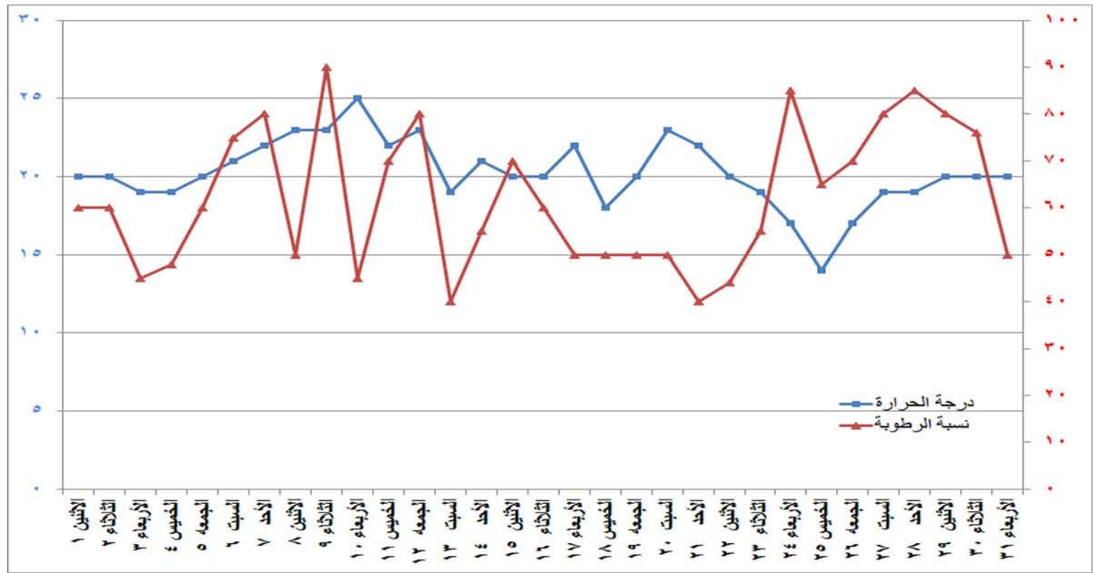
شكل (١١) التغيير في درجة الحرارة والرطوبة النسبية خلال شهر يناير ٢٠١٨
