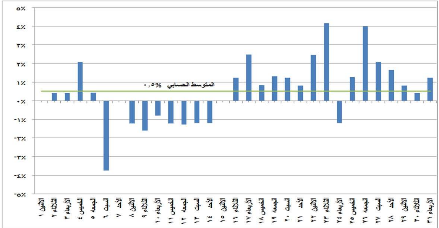
شكل (٩) النسب المئوية للتغير في الحمل الاقصى خلال شهر يناير ٢٠١٨ مقارنة باليوم المماثل من العام الماضي
