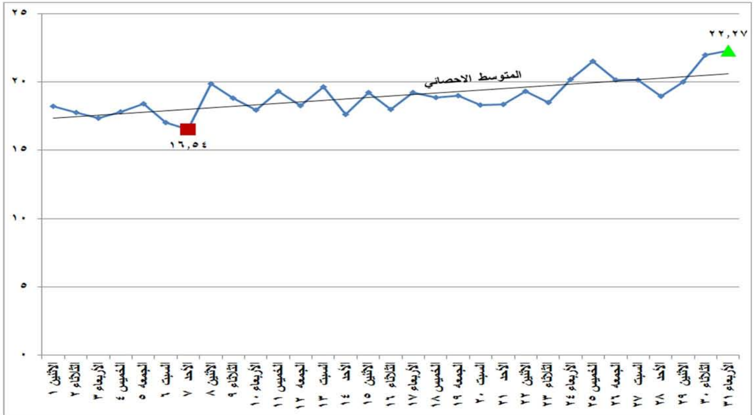
شكل (٢٣) الطاقة الكهربائية المنتجة من المصادر المائية خلال شهر يناير ٢٠١٨
