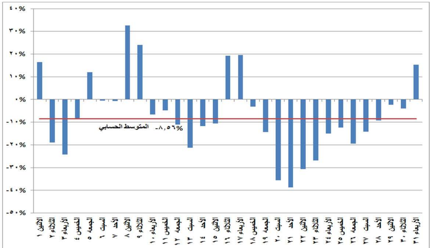
شكل (٢٢) نسب التغير في استخدام المصادر غير الحرارية في إنتاج الطاقة الكهربائية خلال شهر يناير ٢٠١٨ مقارنة بالشهر المماثل من العام السابق
