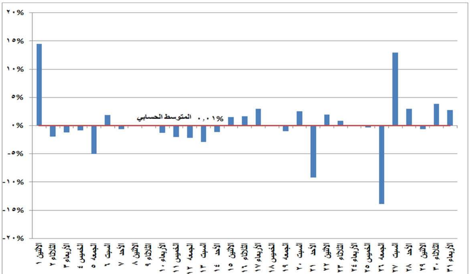
شكل (١٦) نسب التغير في الطاقة الكهربائية المنتجة خلال شهر يناير ٢٠١٨ مقارنة بالشهر المماثل من العام السابق
