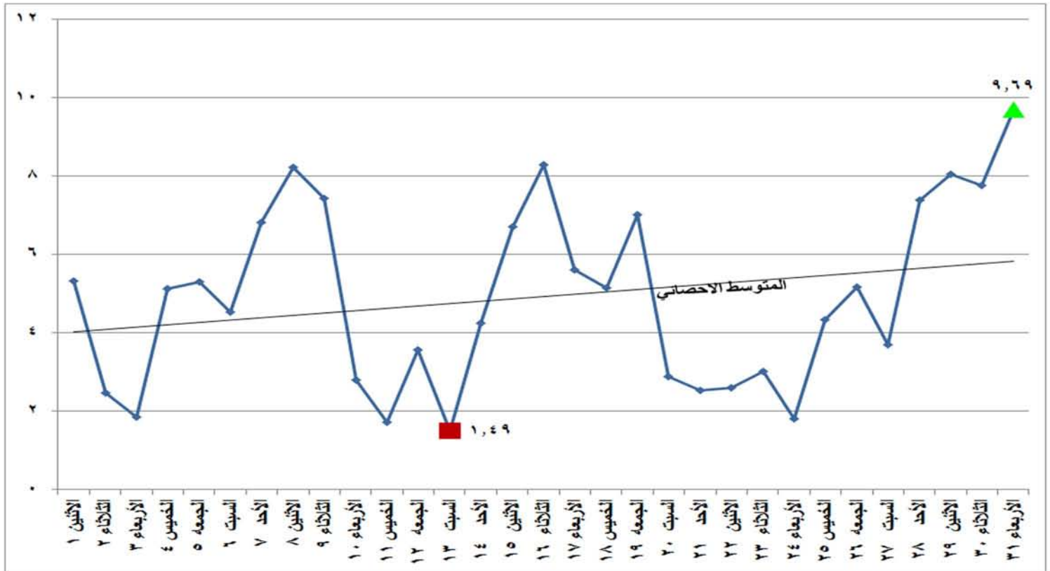
شكل (٢٥) الطاقة الكهربائية المنتجة من الرياح والشمس خلال شهر يناير ٢٠١٨
