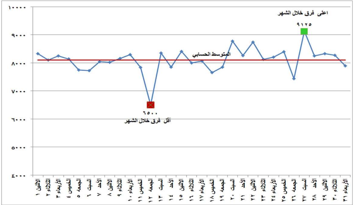
شكل (٣) الفرق بين أقصى وأدنى حمل خلال شهر يناير ٢٠١٨
