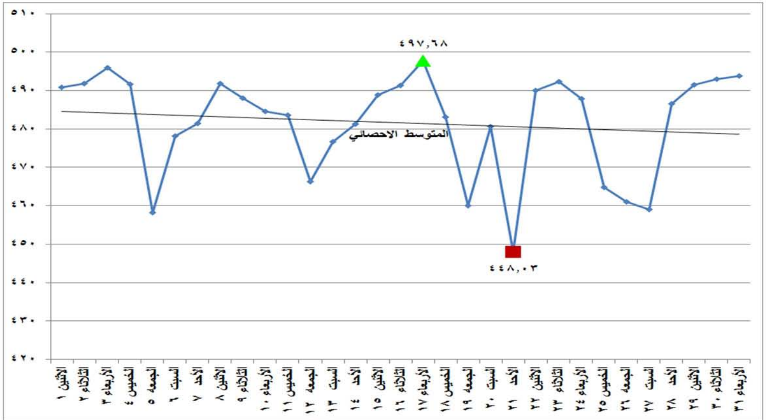
شكل (١٥) أجمالي الطاقة الكهربائية المنتجة من كل المصادر الأولية خلال شهر يناير ٢٠١٨
