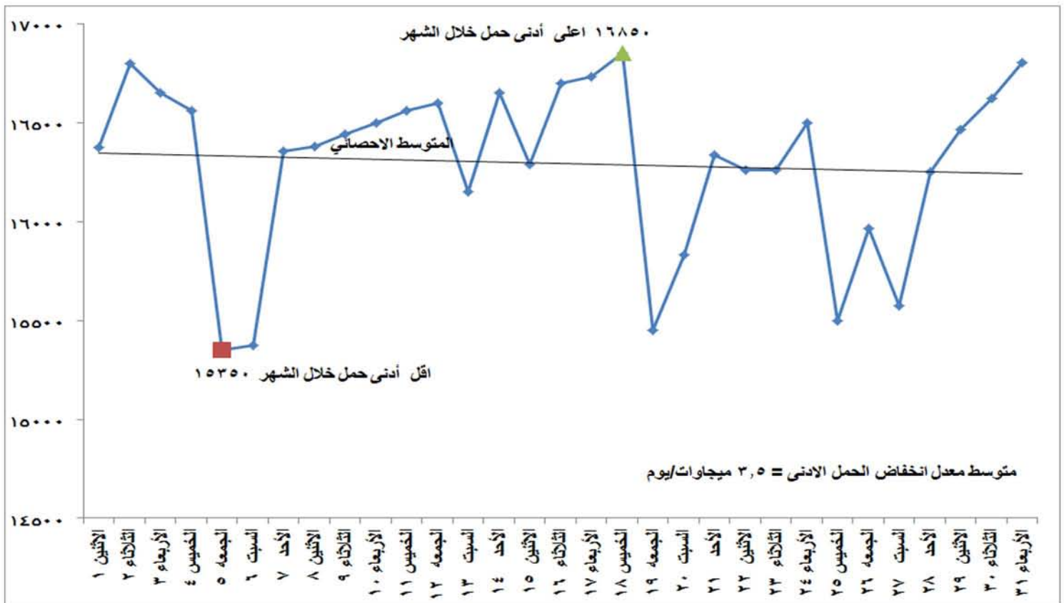
شكل (٢) تطور الحمل الادنى اليومي خلال شهر يناير ٢٠١٨
