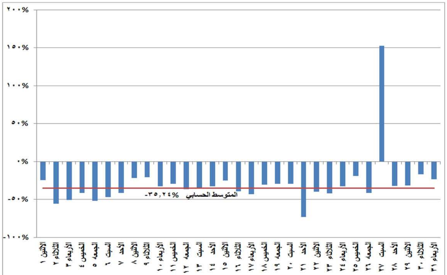
شكل (٢٠) نسب التغير في استخدام المازوت في إنتاج الطاقة الكهربائية خلال شهر يناير ٢٠١٨ مقارنة بالشهر المماثل من العام السابق
